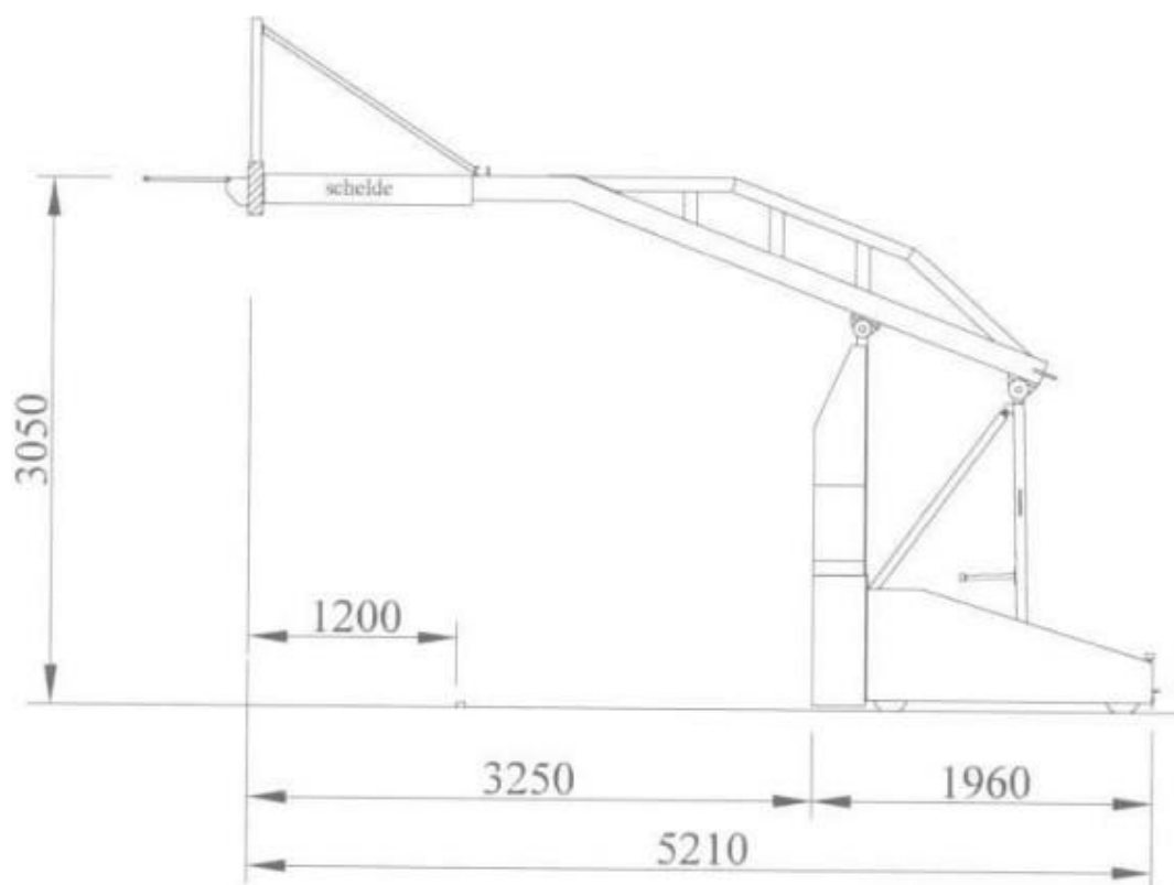
Zijaanzicht
